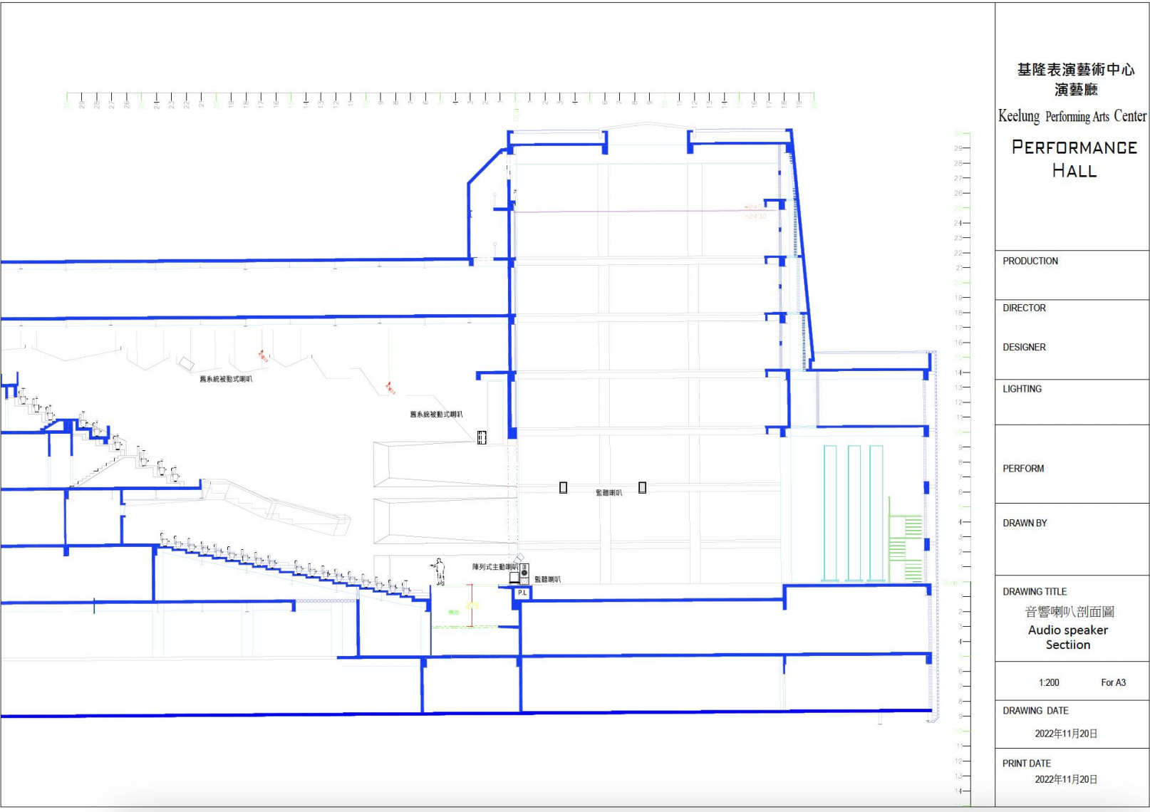
音響喇叭位置剖面圖
